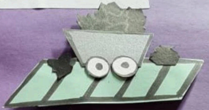
فحم حجري
